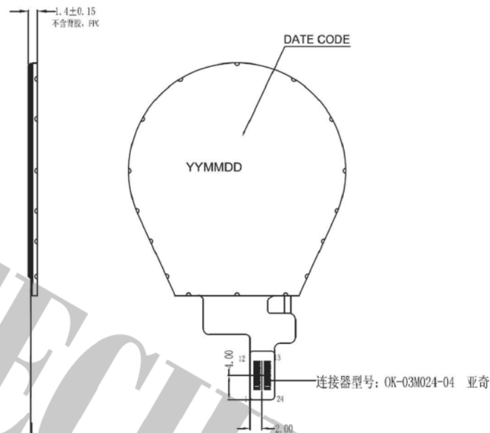
FPC弯折示意图 FPC展开出货
