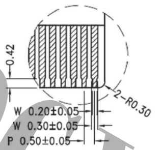
Detail a Scale: 5X
